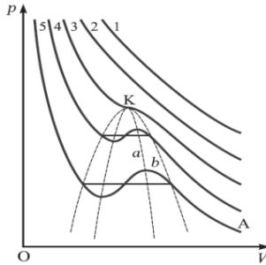
Նկ. 1. Վանդերվաալ սյան գազի իզոթերմերի ընտանիք:
