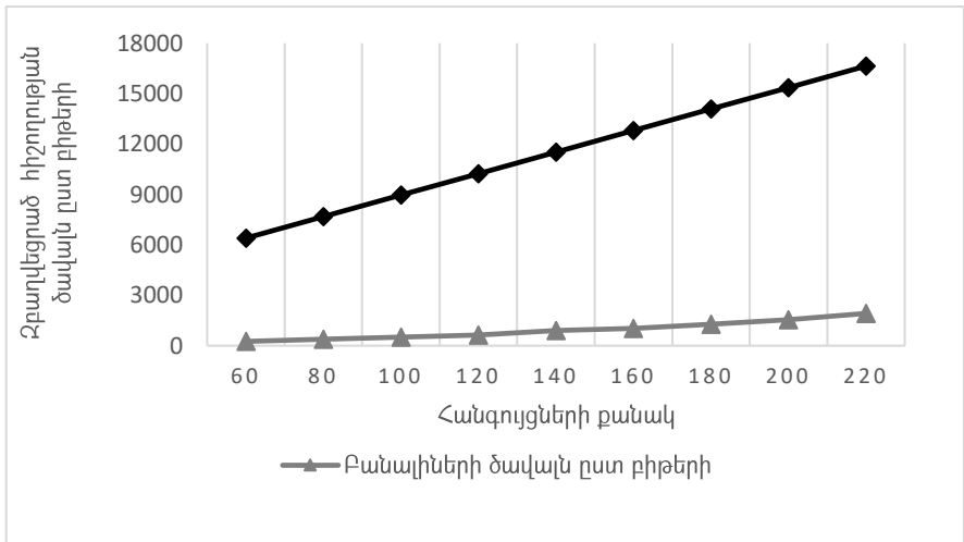
Նկ.3. Բանալիների պահպանման համար անհրաժեշտ հիշողության ծավալի համեմատականը դասական և առաջարկված մեթոդների դեպքում
