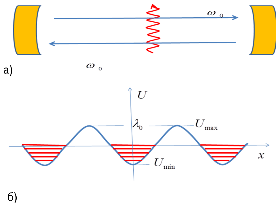
Рис. 3. Схематическое представление ЛСЭ со стоячей электромагнитной волной (а) и эффективная потенциальная энергия электрона в поле стоячей волны (б) .
