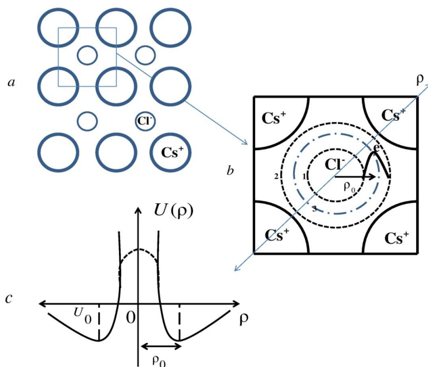
Рис.7. а) Решетка кристалла CsCl , б) ячейка решетки , в) эффективный потенциал каналирования позитронов вокруг оси отрицательно заряженных ионов Cl^- показан вдоль радиуса \rho , который в области локализации позитрона описывается потенциалом Морса.
